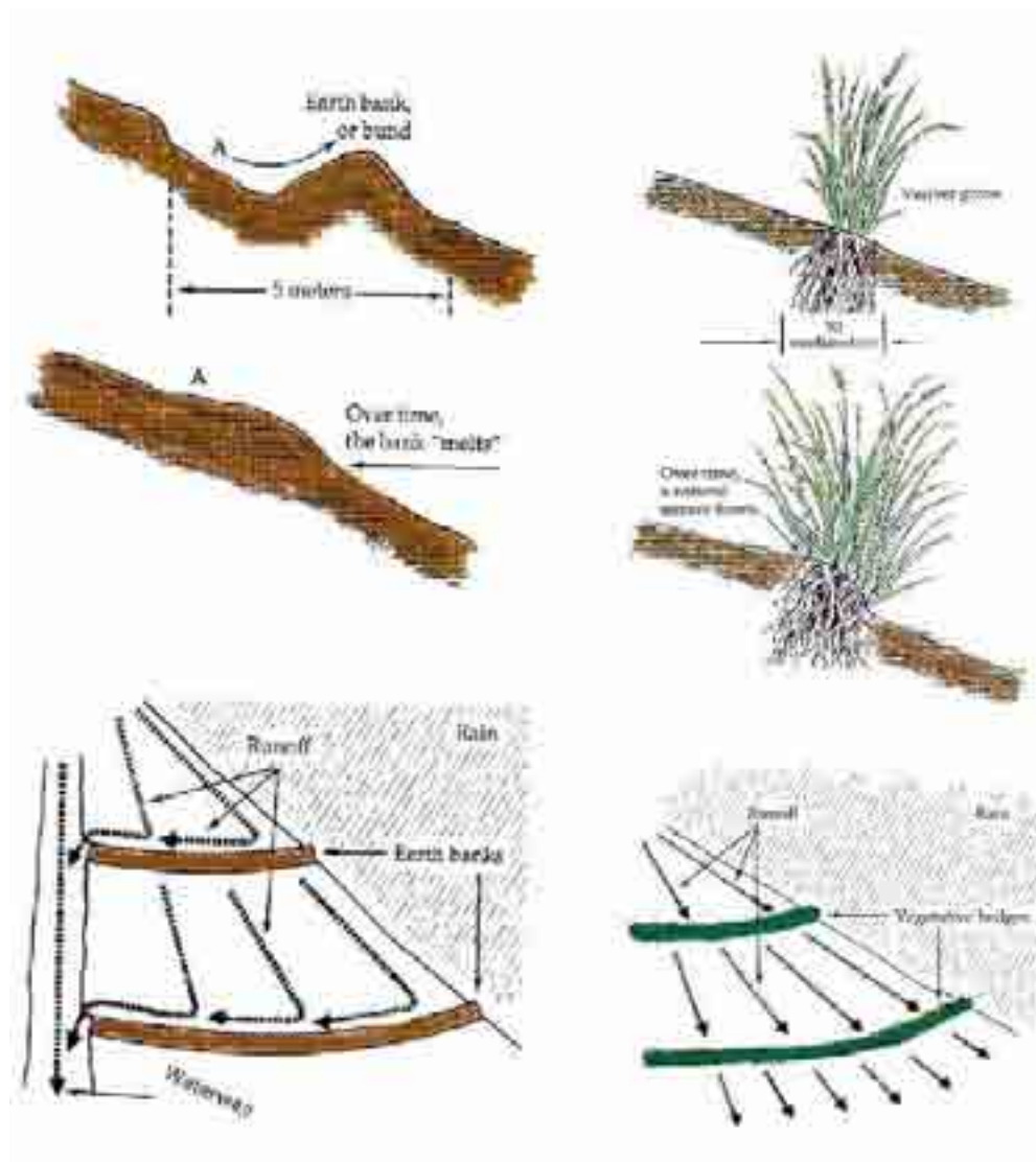
Hình 1: Bờ đất đắp theo đường đồng mức trên sườn dốc (trái trên) góp phần lái dòng chảy ra nơi khác (trái dưới). Hàng rào cỏ Vetiver dần dần cũng tạo nên các bờ đất (phải trên) nhưng vẫn cho nước mặt chảy chậm và dàn đều trên sườn dốc (phải dưới), qua đó giảm nhẹ rửa trôi, xói mòn và nước mặt ngấm nhiều hơn, sâu hơn xuống dưới đất (Greenfield 1989).
