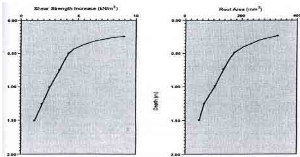
Hình 3: Tác dụng tăng sức kháng cắt của rễ cỏ Vetiver theo chiều sâu đất
