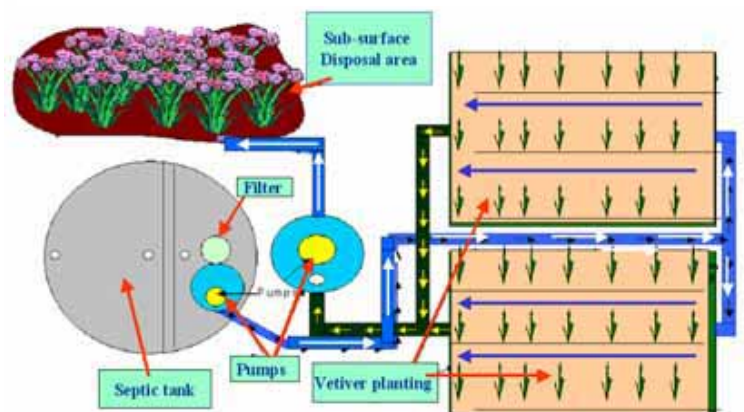
Hình 5: Sơ đồ bố trí xử lý nước thải sinh hoạt bằng cỏ Vetiver.
