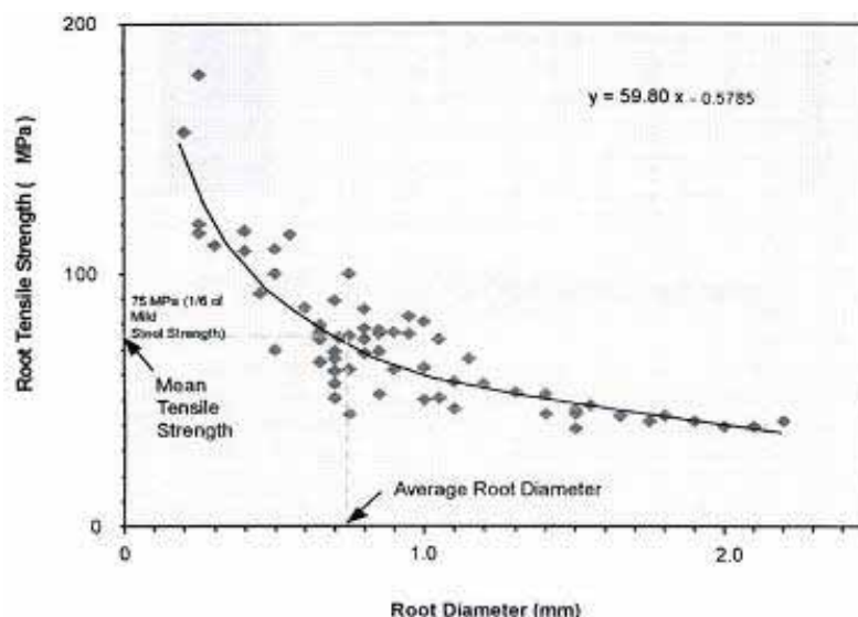
Hình 2: Tương quan sức kháng kéo - đường kính rễ cỏ Vetiver
