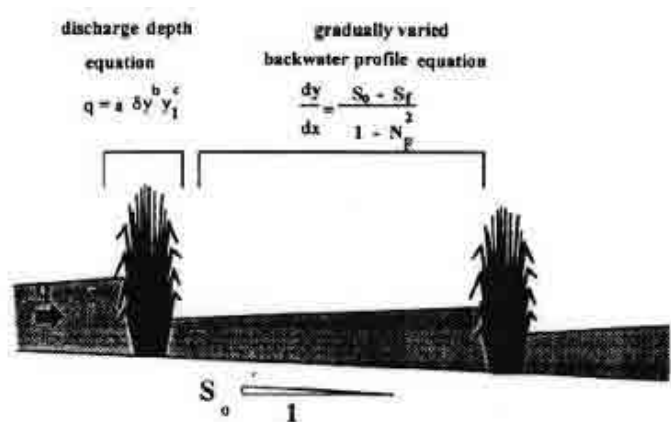
Hình 4: Mô hình thủy lực giảm nhẹ cường độ lũ bằng các hàng cỏ
