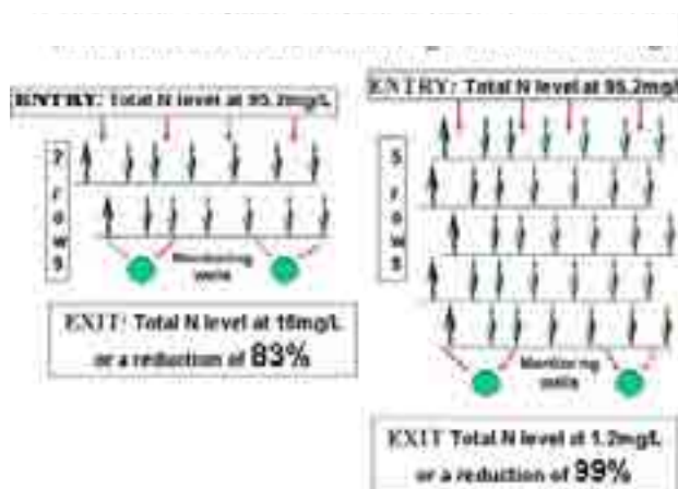
Hình 4: Hiệu quả của cỏ Vetiver tiêu giảm Nito trong nước thải sinh hoạt
