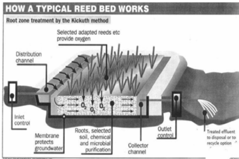
Hình 6: Mô hình lọc nước thải bằng các luống cỏ Vetiver
