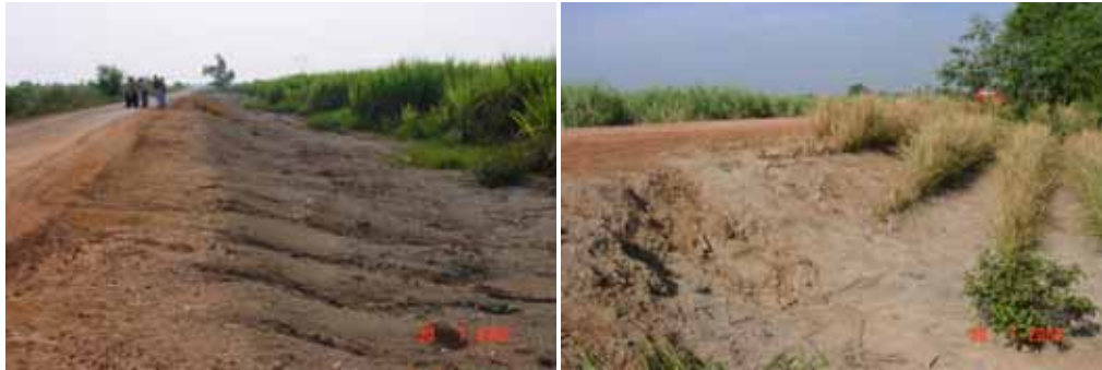
Ảnh 21: Nền đường trên đất chua phèn nặng ở Tiền Giang trước và sau khi trồng cỏ Vetiver.
