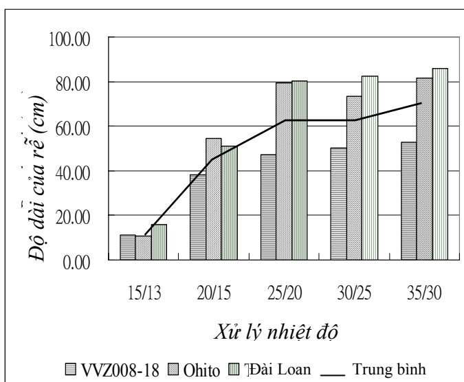
Hình 2: Ảnh hưởng của nhiệt độ đất tới khả năng phát triển rễ cỏ Vetiver
