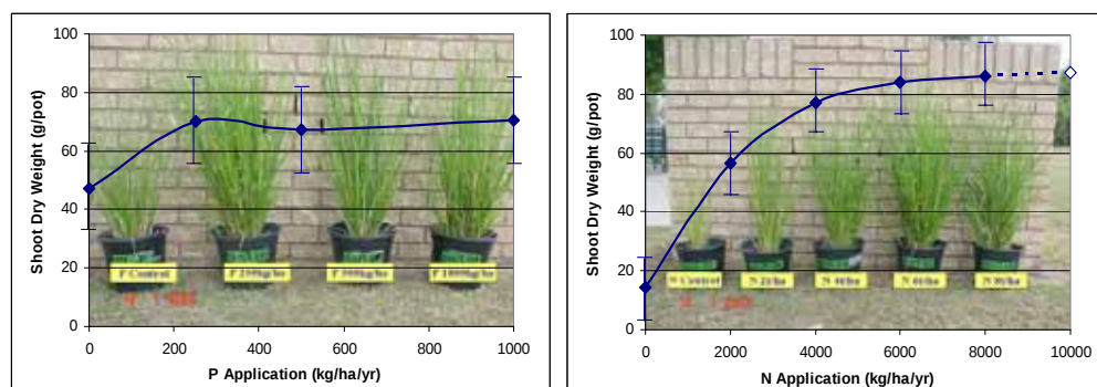
Hình 2: Khả năng hấp thụ và chịu được nồng độ N và P cao
